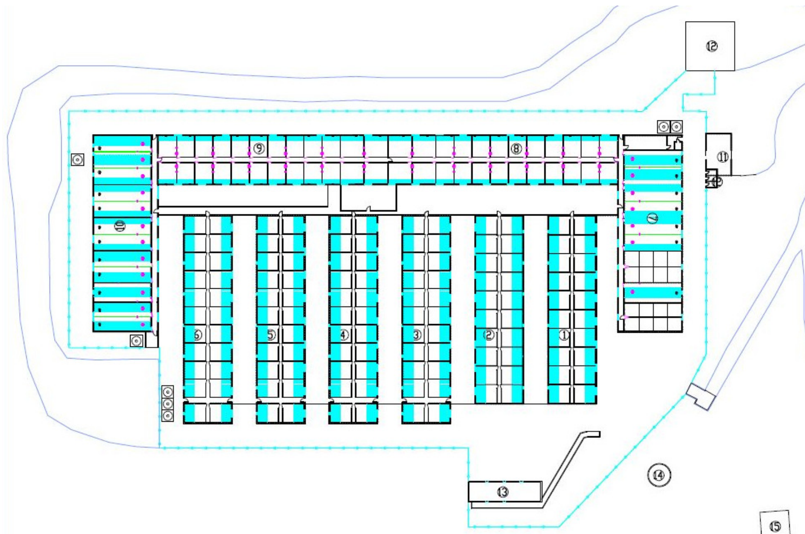
Planta Sínte da Instalação Suinícola "Mirante".
